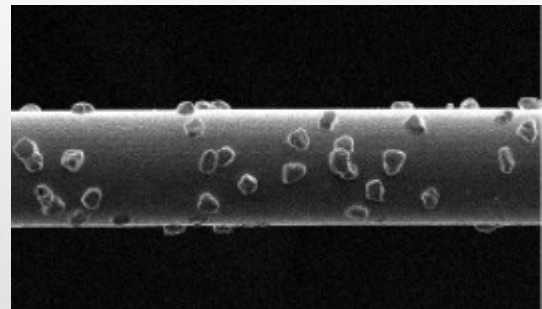
製品写真（芯線径Φ80、砥粒径Φ10）
