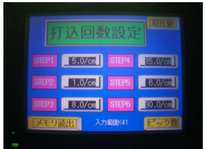
打込回数 設定画面
