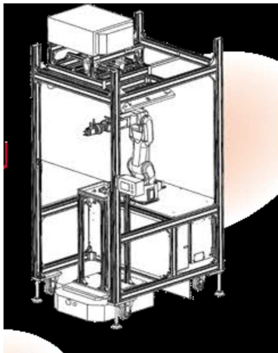
弊社で過去に製作したロボットを活用した生産設備の一例 (3次元ビジョンセンサを用いたばら積みピッキング装置デモ機)
