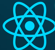
React.js
