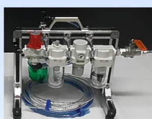
操作盤（3） エア4点セット
