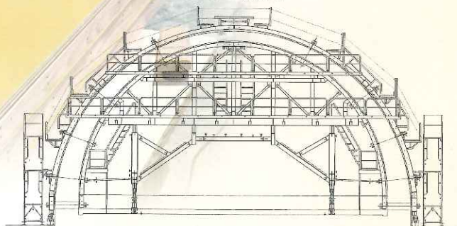
トンネル 断面図
