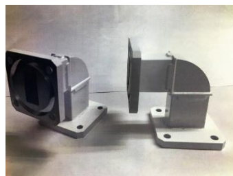
L字導波管
