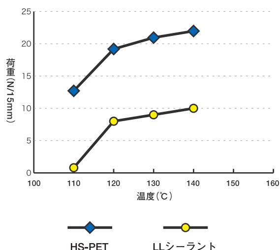
HS-PET & LLシーラント熱傾斜比較
