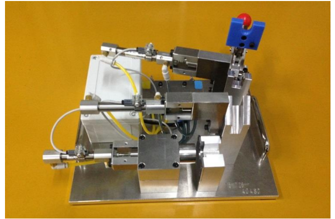
パイプ寸法検査治具 Pipe size inspection jig
