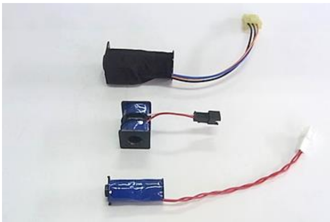
ソレノイドコイル Solenoid coil
