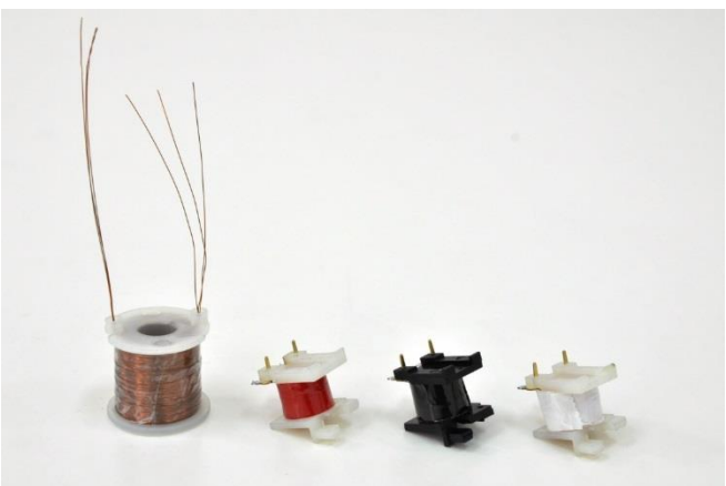
リレーコイル Relay coil
