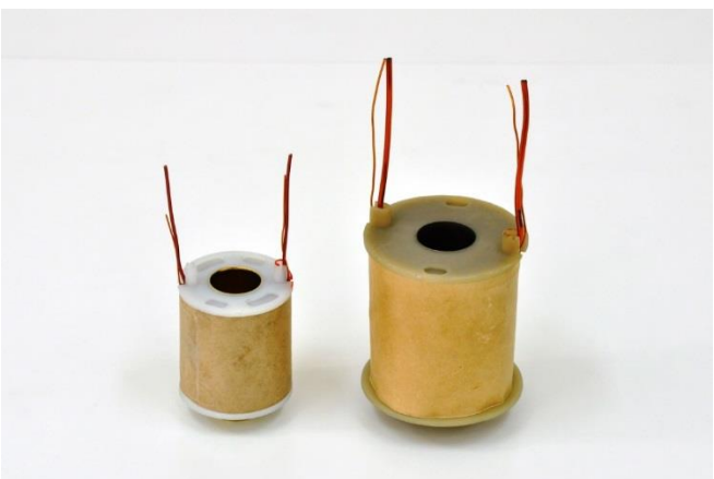
エンジンスターター用コイル Engine starter coil
