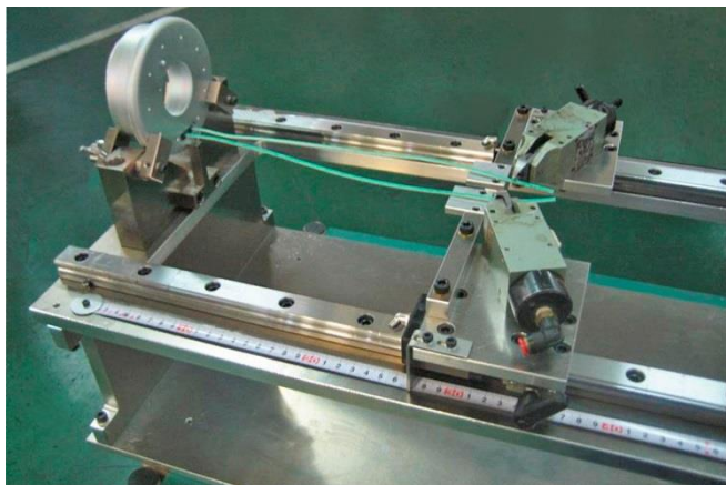
コードカット治具 Cord cutting jig
