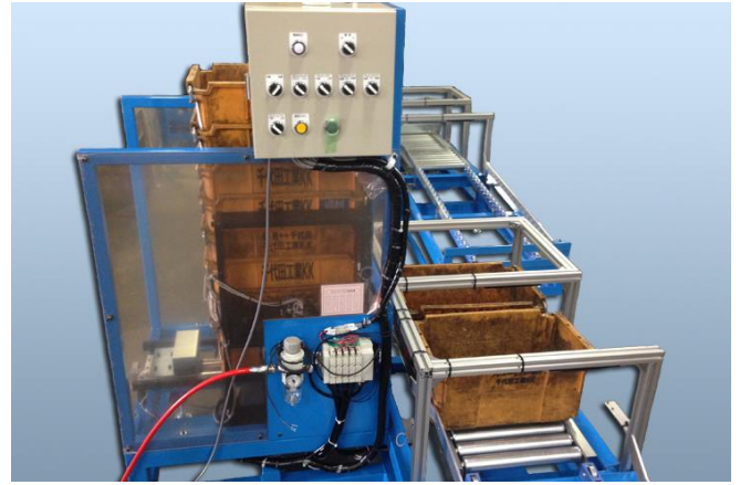
パレットチェンジャー Pallet changer
