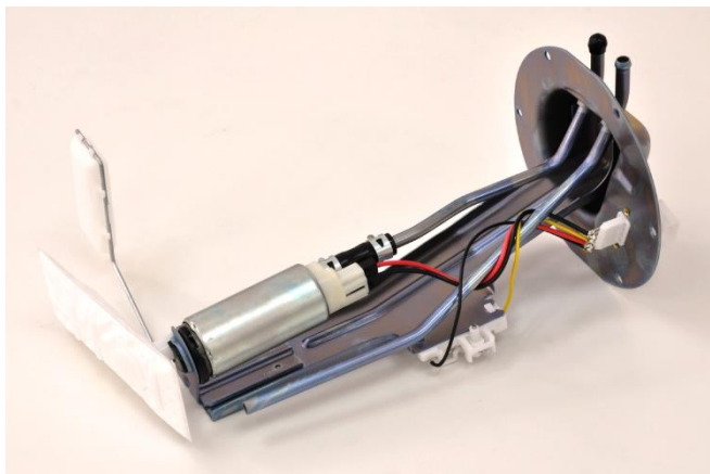
自動車用燃料ポンプユニット Fuel pump unit for vehicle
