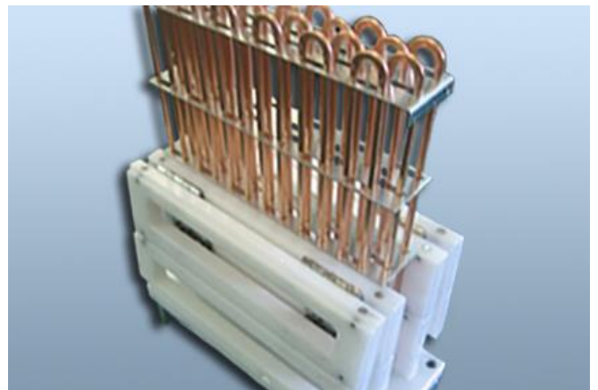
フィン挿入治具 Fin insert jig
