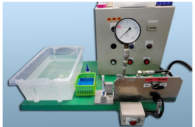
パイプ漏洩検査機（水没式） Submerge type leakage inspection device
