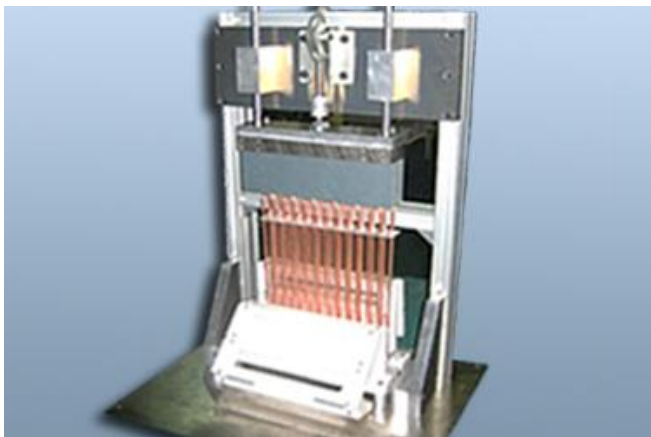
フィン挿入装置 Fin inserter
